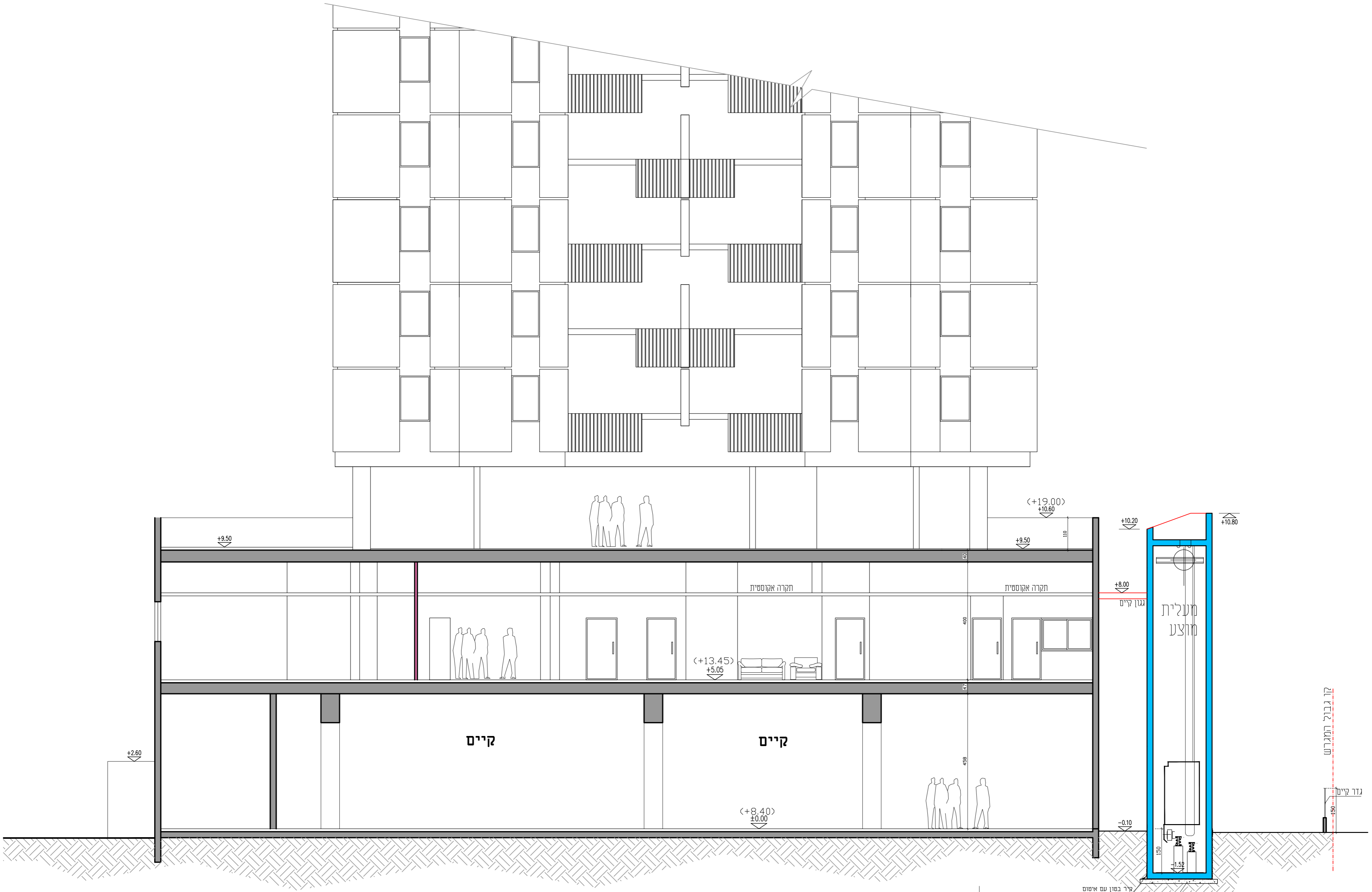
צתך 2-2 קני"מ 1:100
